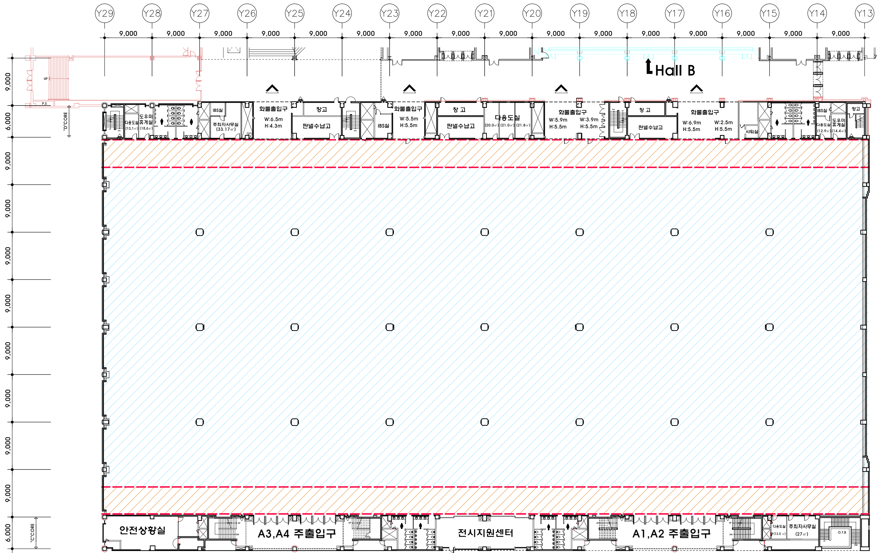
1F Hall A 천장평면도
