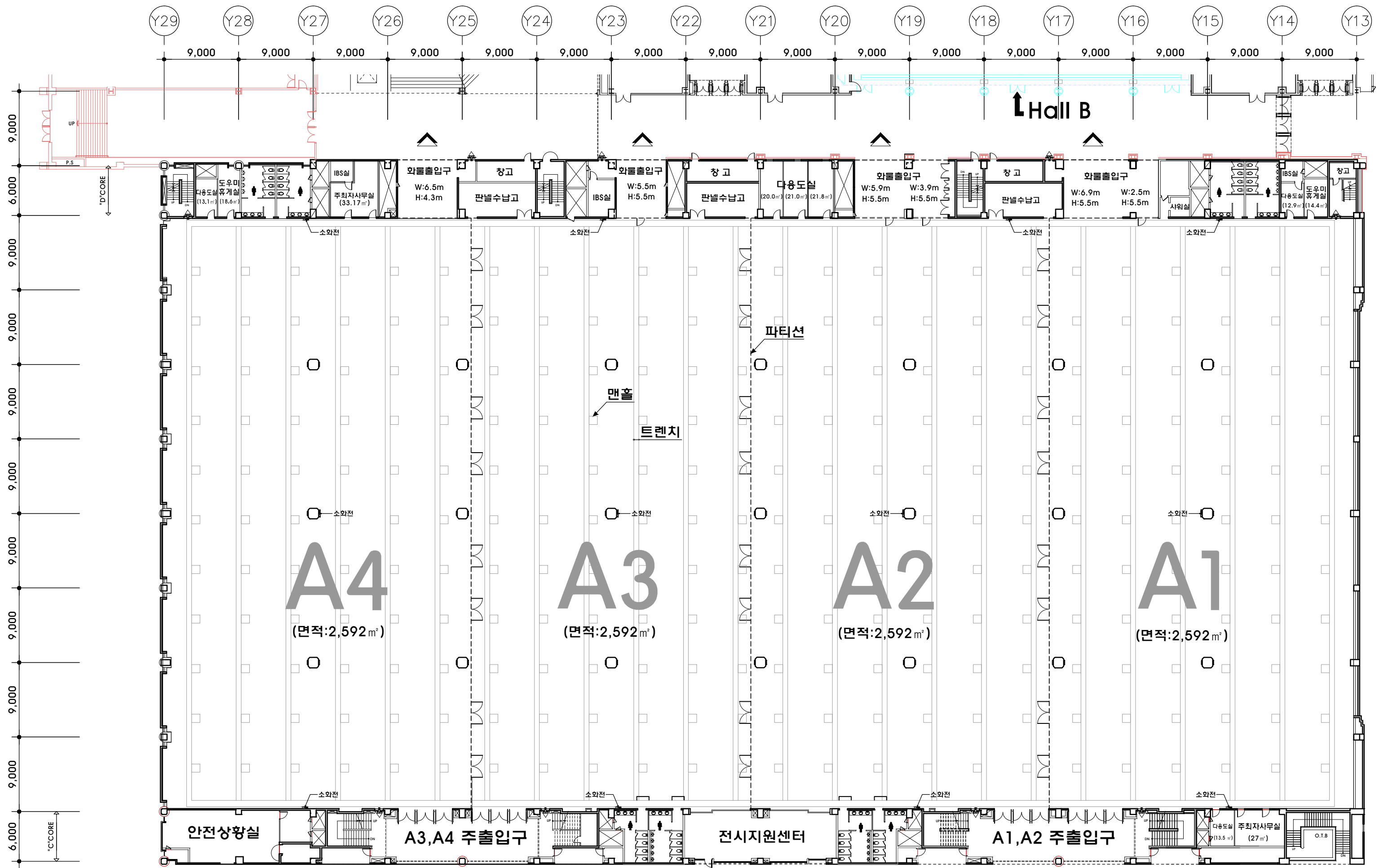
1F Hall A 평면도
